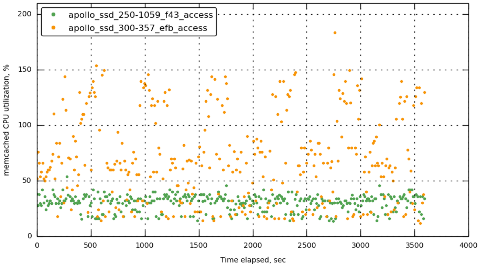
[172.23.96.16] memcached_cpu
