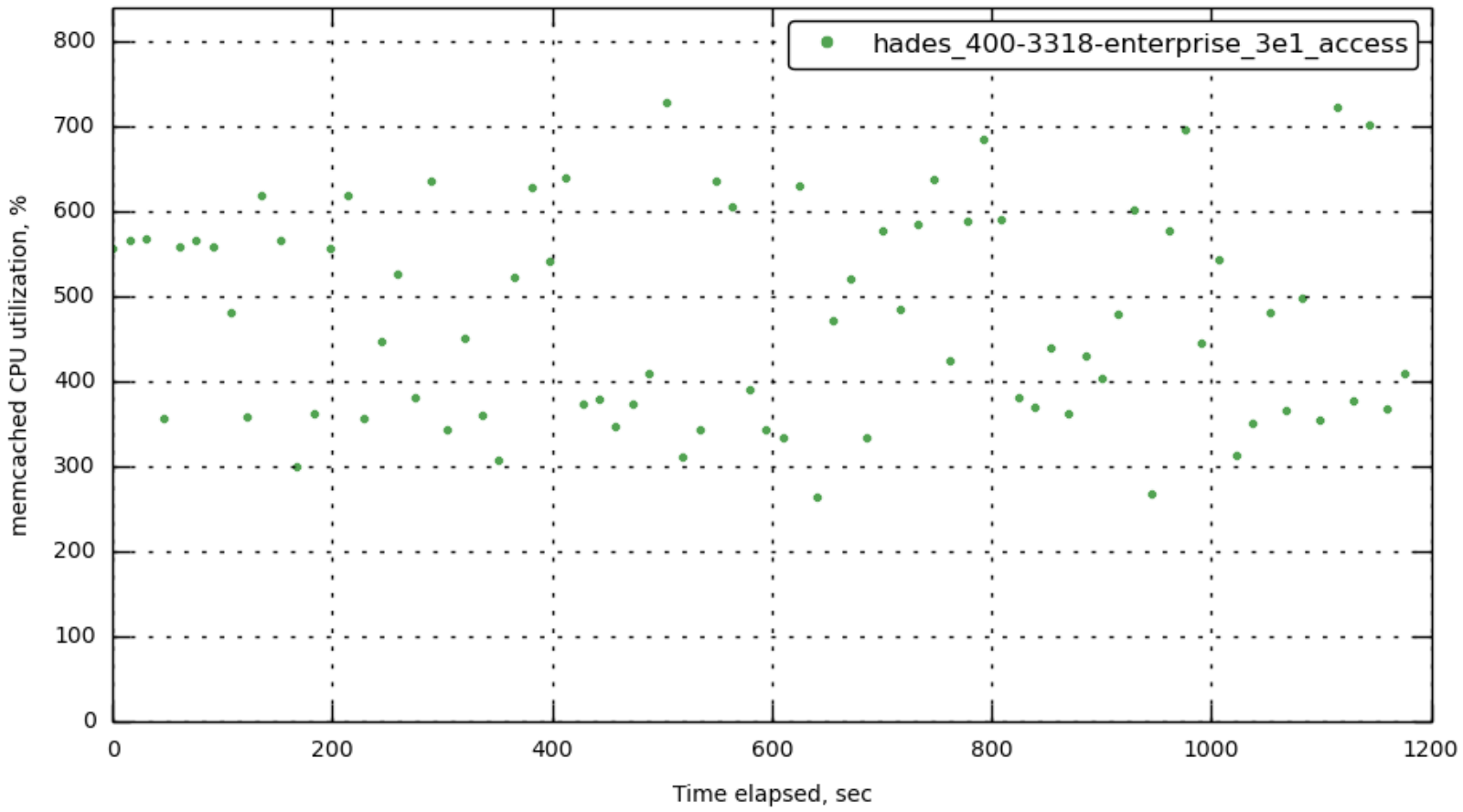
[172.23.100.71] memcached_cpu
