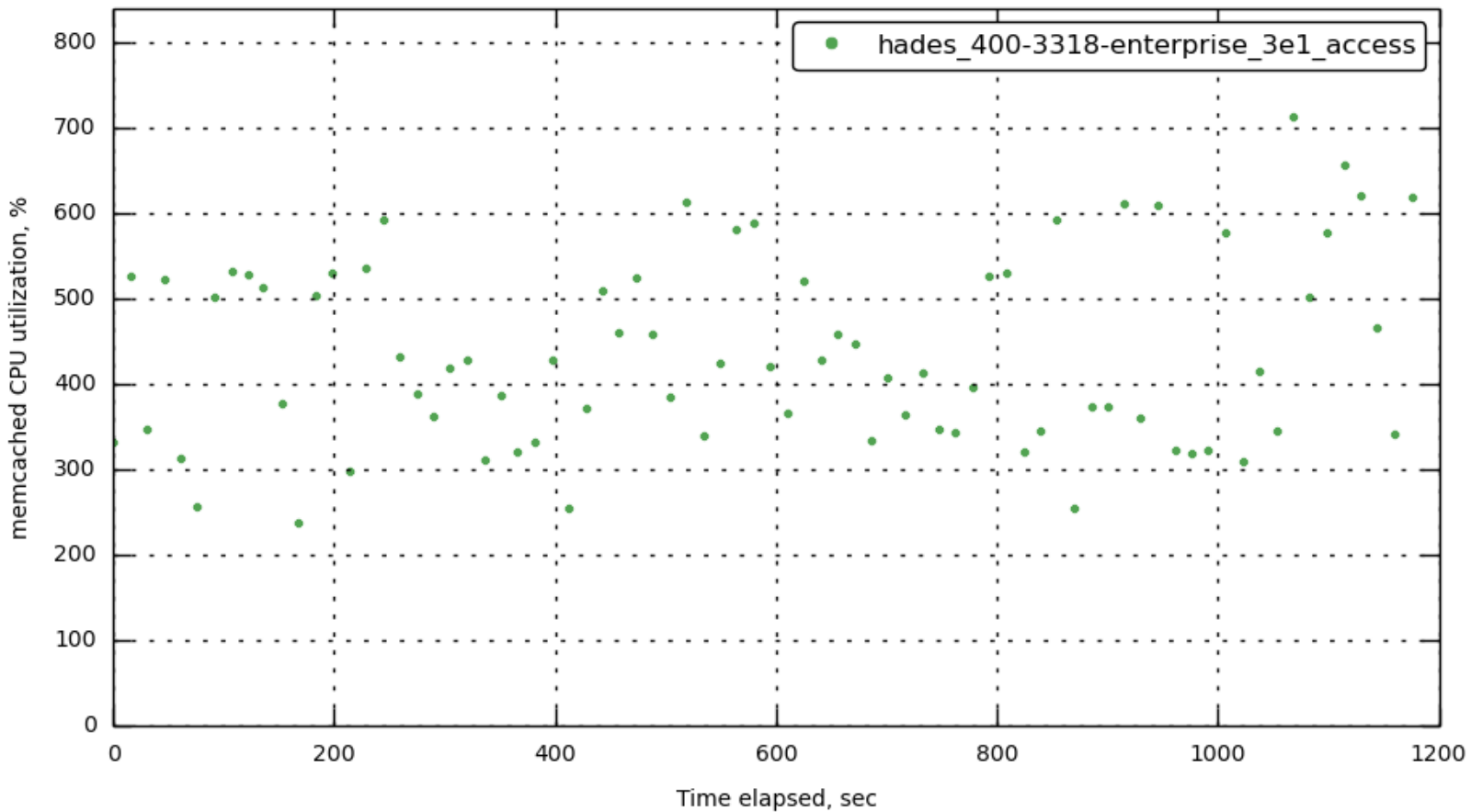
[172.23.100.72] memcached_cpu
