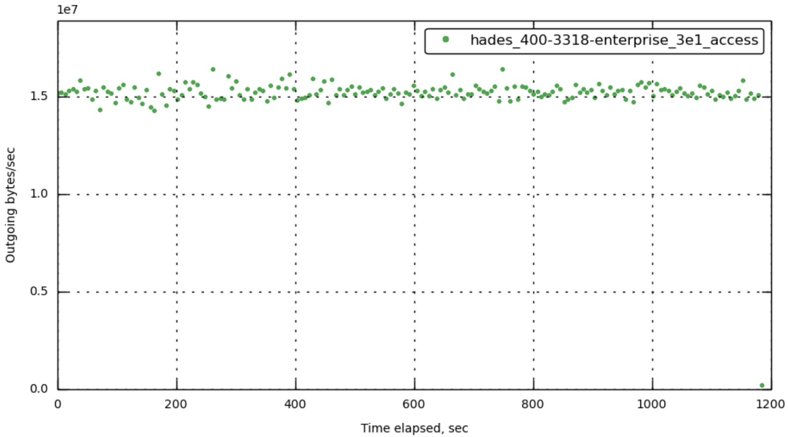
[172.23.100.72] out_bytes_per_sec
