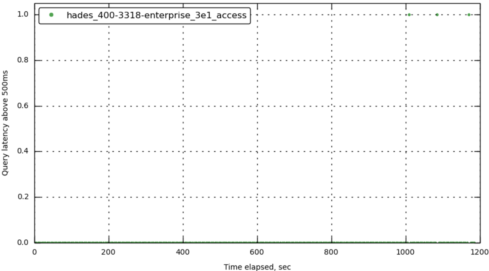
query_requests_500ms
