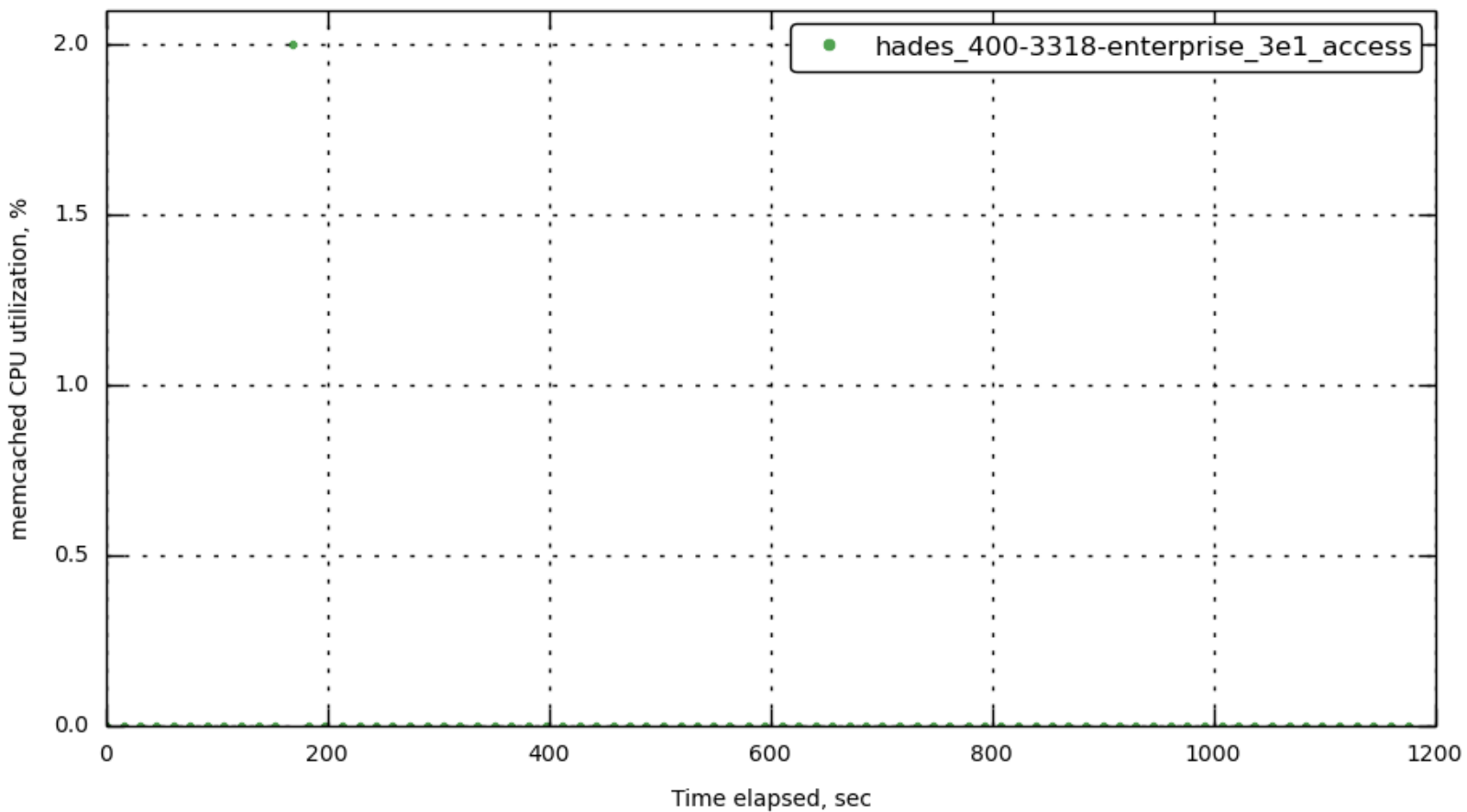
[172.23.100.45] memcached_cpu
