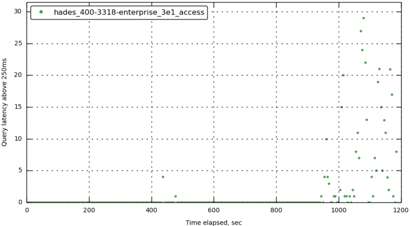
query_requests_250ms
