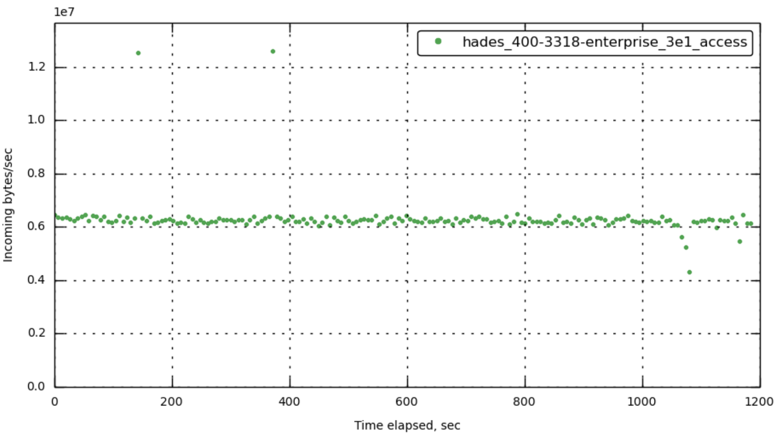
[172.23.100.55] in_bytes_per_sec
