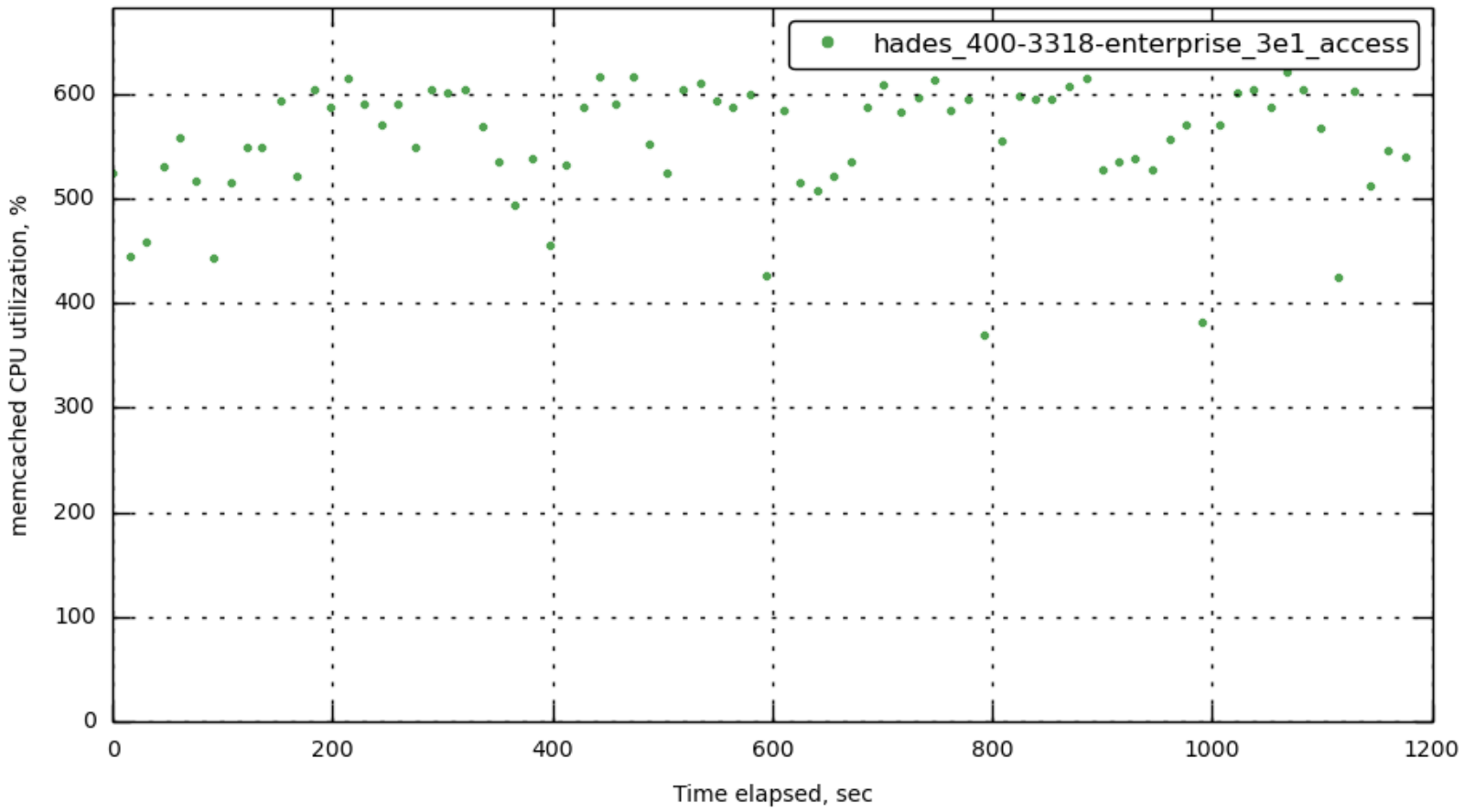
[172.23.100.73] memcached_cpu
