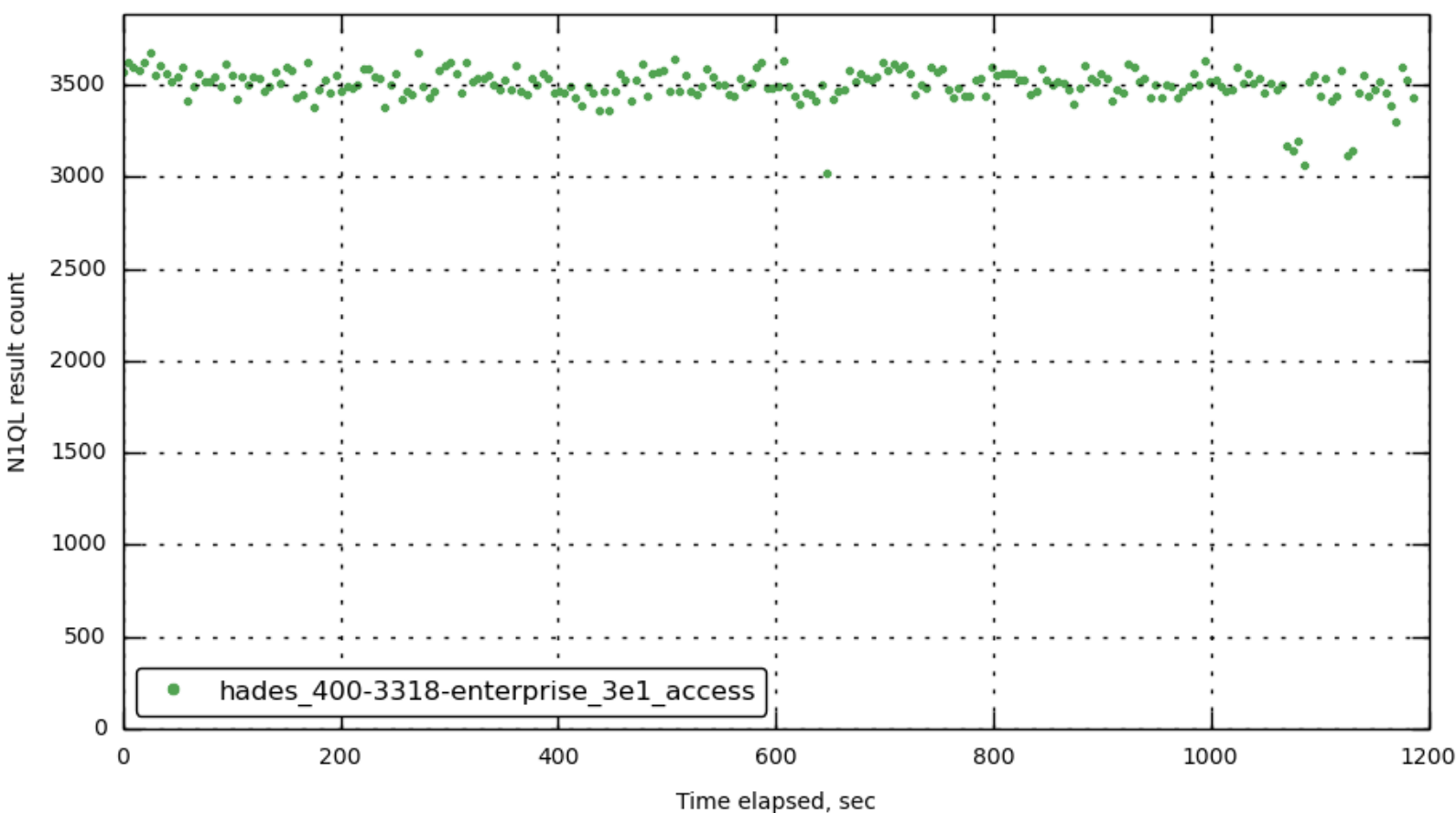
query_result_count
