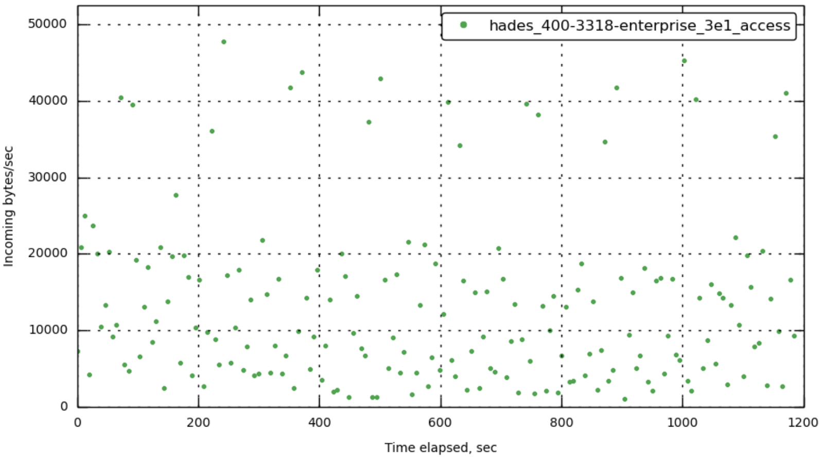
[172.23.100.45] in_bytes_per_sec
