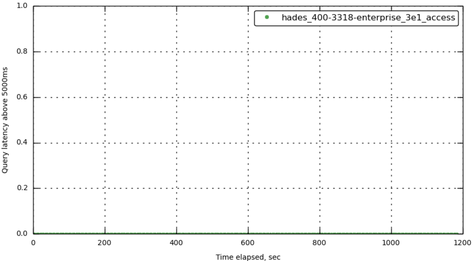
query_requests_5000ms
