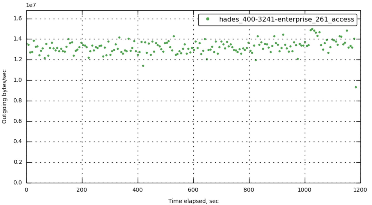
[172.23.100.72] out_bytes_per_sec
