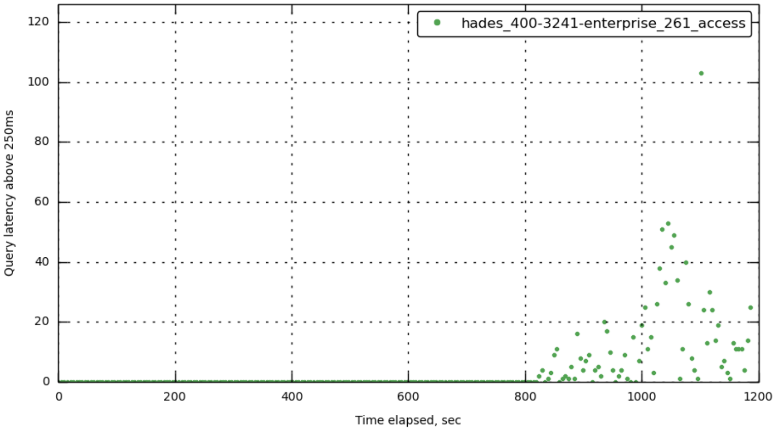
query_requests_250ms
